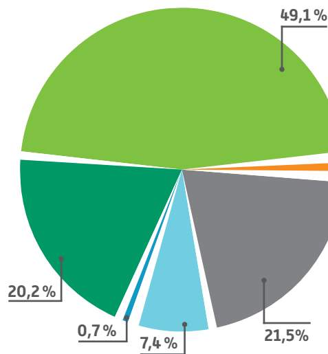
verbleibender Energieträgermix
